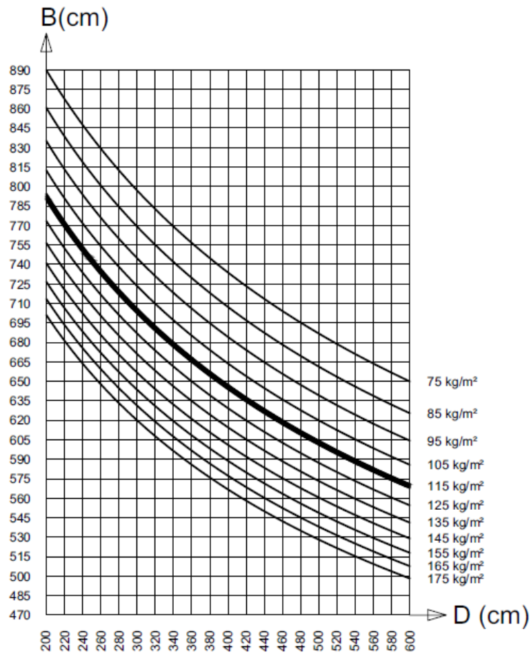
Bild 2: Statiktabelle mit Staleinschub
