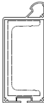
Bild 2: Statiktabelle mit Staleinschub
