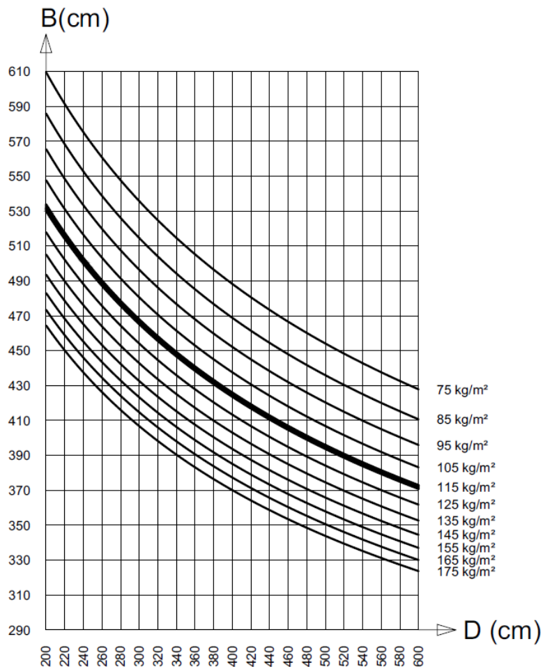
Bild 1: Statiktabelle ohne Staleinschub
